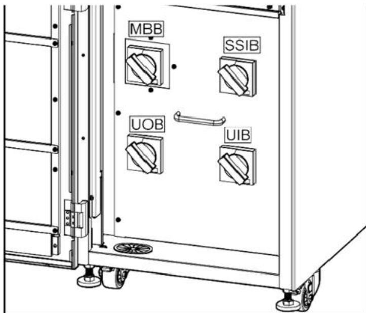
Рисунок 10-4. ИБП мощностью 60 кВА 400 В с внутренними батареями, вид спереди
