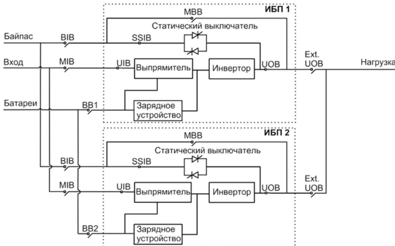
Рисунок 13-1. Параллельная система с резервированием 1+1 с общим батарейным массивом
