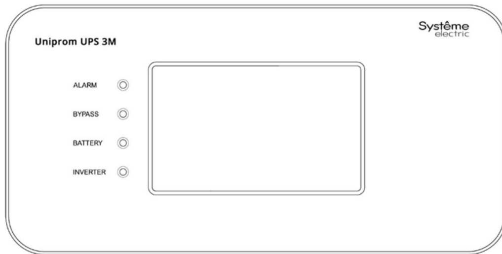
Рисунок 7-1. Пользовательский интерфейс
